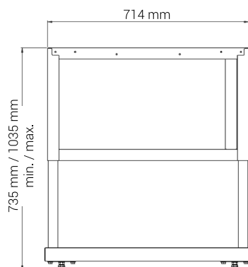
Adjustable stand
