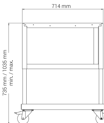
Adjustable stand
