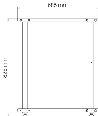
Fixed stand
